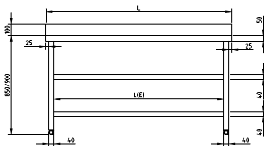
ALZADO
